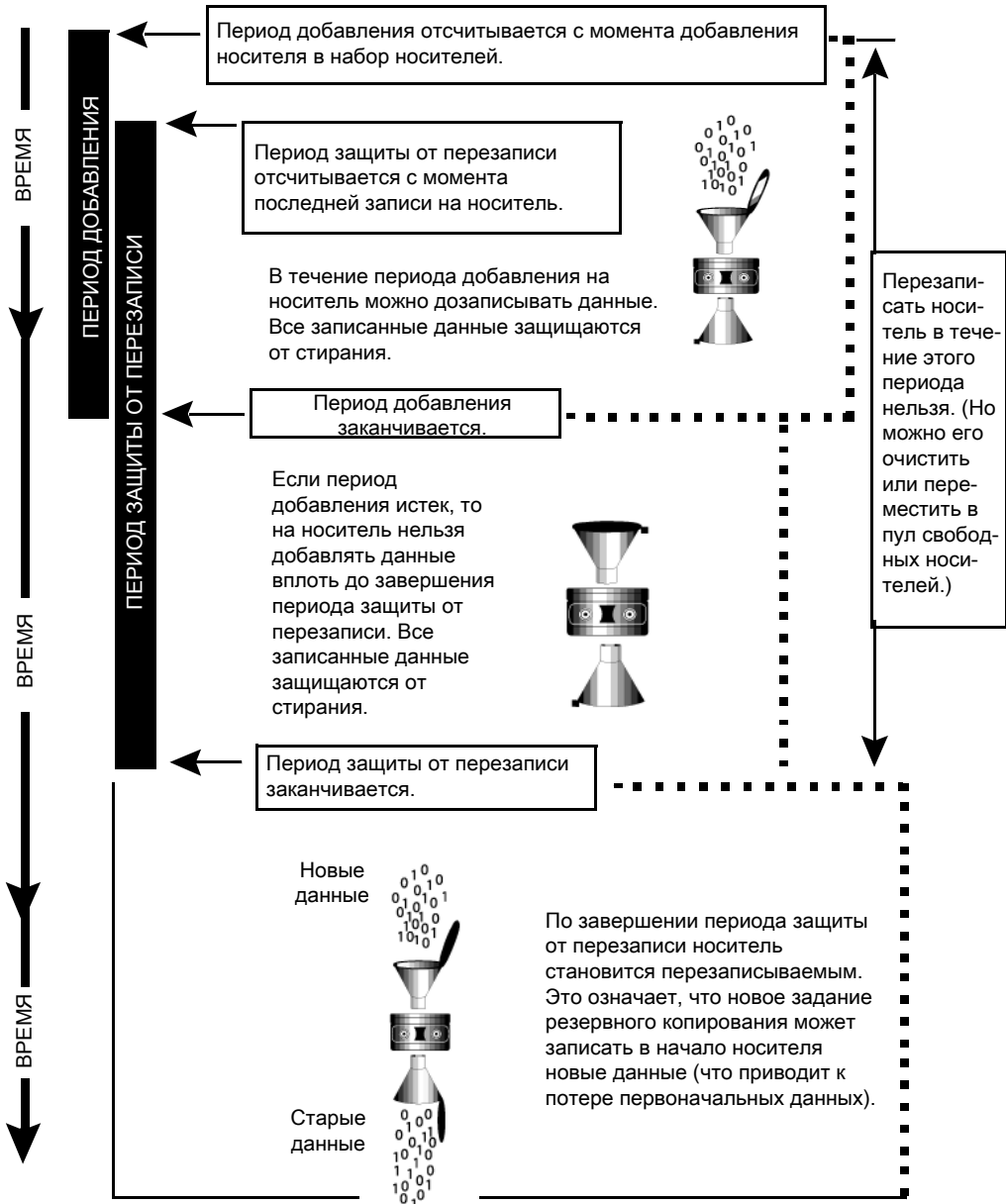
Рис. 10-1 Периоды добавления и периоды защиты от перезаписи
