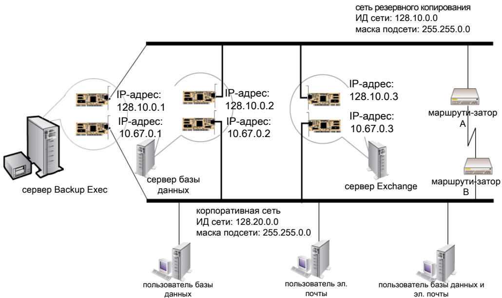
Рис. 14-1 Пример сети резервного копирования
