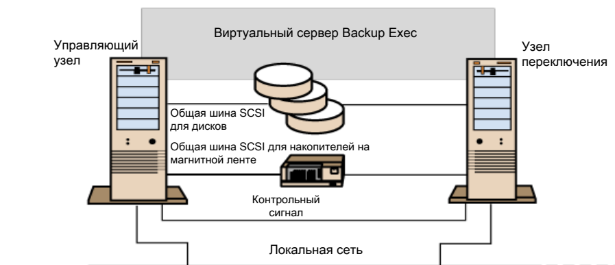
Рис. 17-2 Кластер, состоящий из двух узлов, с накопителями на магнитной ленте на общей шине SCSI
