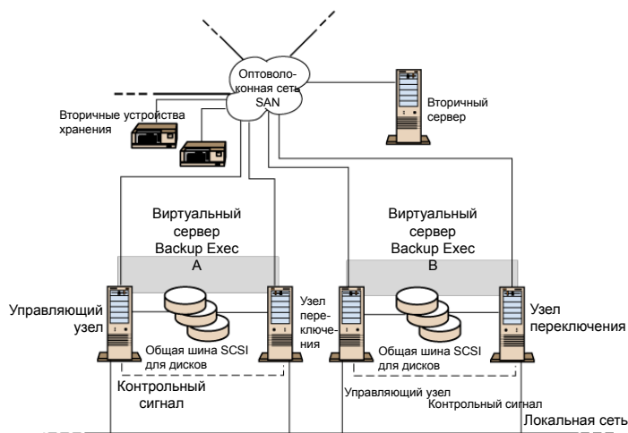
Рис. 17-3 Пример общей шины с накопителями на магнитной ленте в конце шины
